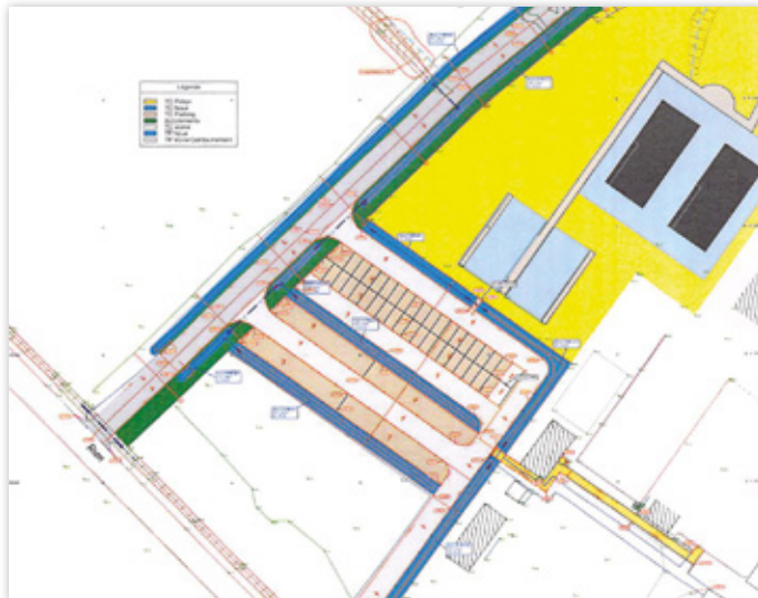
Plan montrant la nouvelle voirie de contournement.
